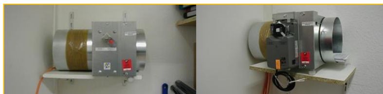
Clapets coupe-feux à réarmements manuels ou motorisés
